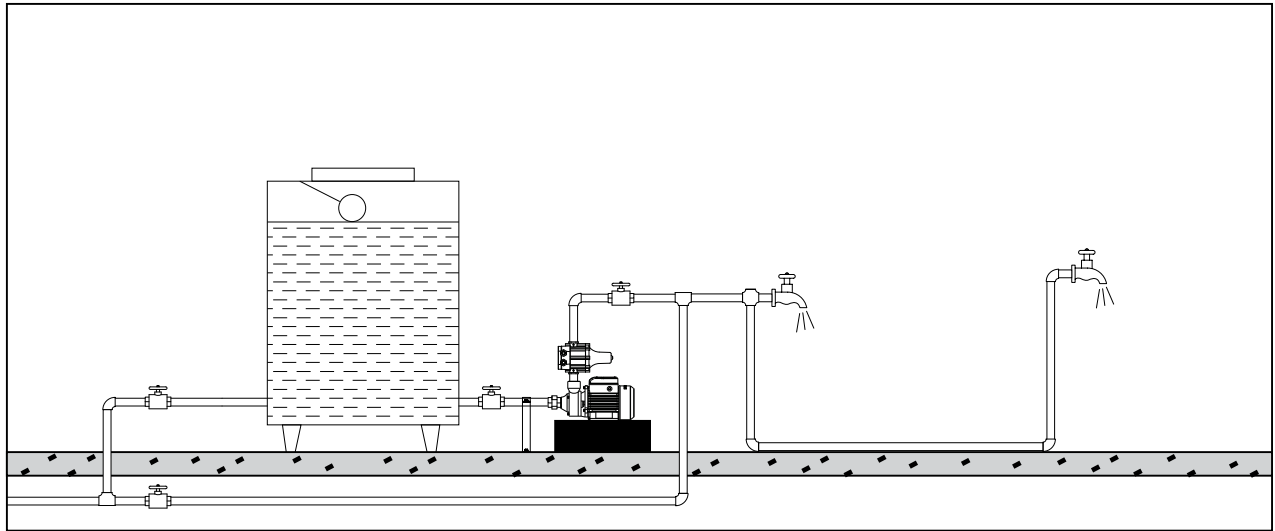
Presurización de agua de grifo o aspersores
